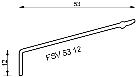
Fensterschienen Verbreiterung für FS 16 42
