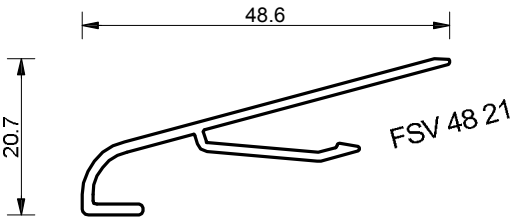
Fensterschienen Verbreiterung für FS 48 21
