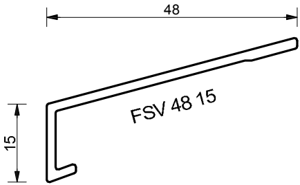
Fensterschienen Verbreiterung für FS 24 41
