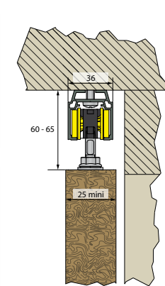
Fixation plafond
