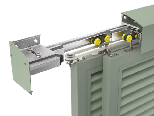
- 2 vantaux en double voie
