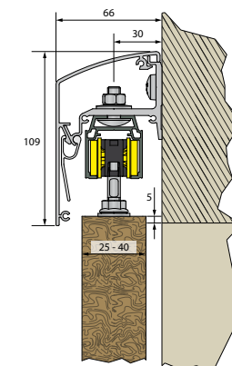
Fixation murale 1 voie
