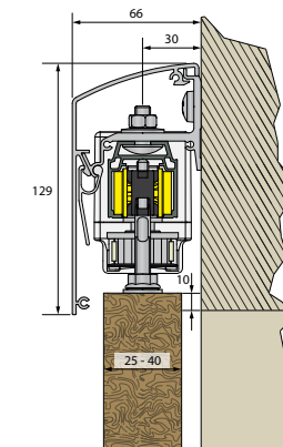
Fixation murale 1 voie motorisée
