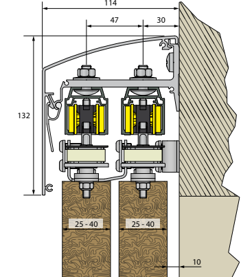
Fixation murale 2 voies synchronisées
