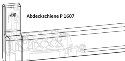
Abdeckkappe 9-38542-00-L-*
