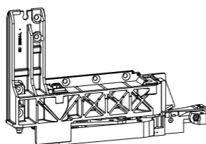
Laufschuh vorn li. 6-32544-00-L-0 re. 6-32544-00-R-0
