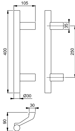
Aluminium-Stützen Edelstahl-Stange
